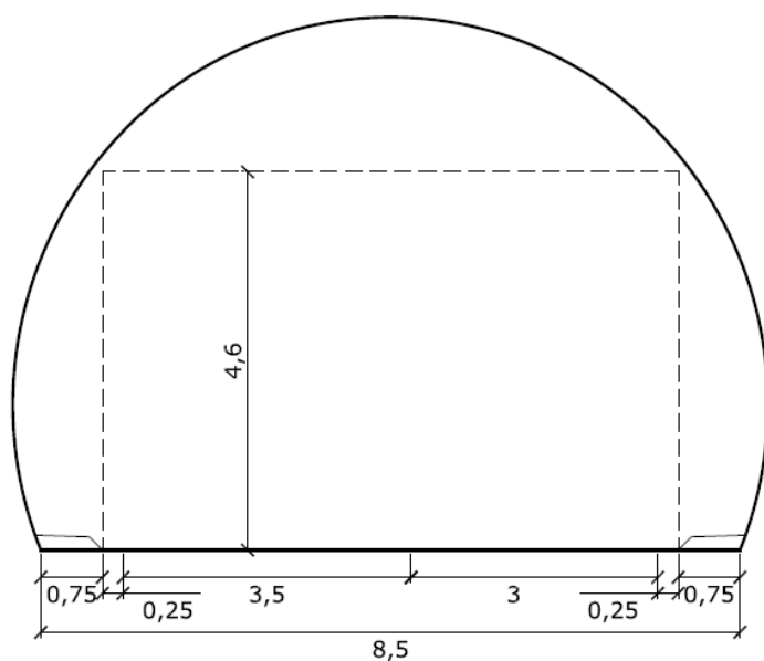
Figur V1.16 Tunnelprofil T8,5 med møteplass (mål i m).
