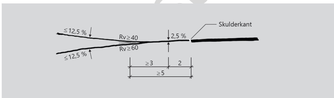
Figur D.24: Krav til vertikal linjeføring i avkjørsler (mål i m)
