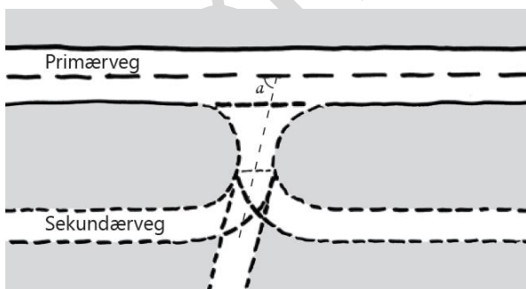
Figur D.1: Standardisert utforming av sekundærvæg
