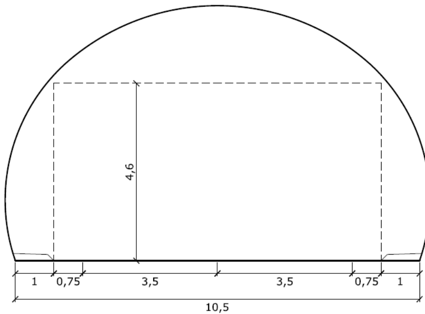
Figur V1.8 Tunnelprofil T10,5 (mål i m).
