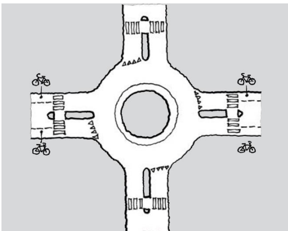
Figur D.13: Prinsippløsning for sykkel i rundkjøring, eksempel 1
