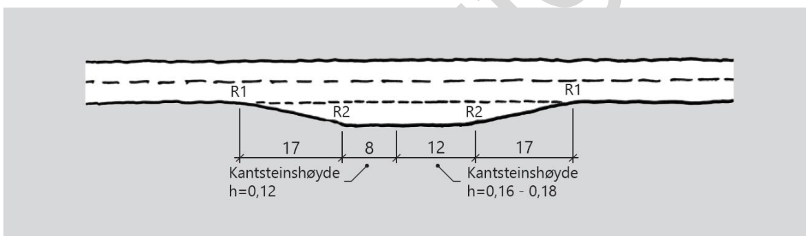
Figur D.39: Busslomme ved utbedringsstandard (mål i m)
