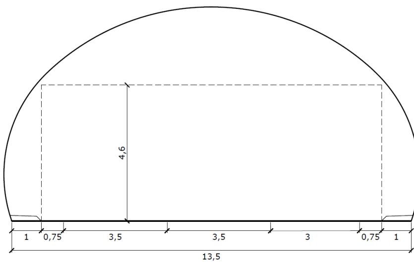
Figur V1.9 Tunnelprofil T13,5 med havarilomme (mål i m).
