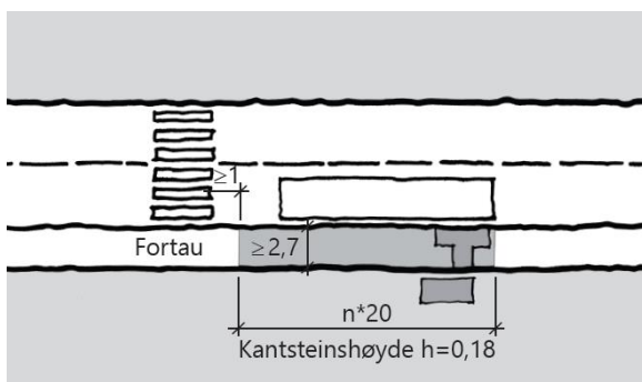
Figur D.36: Kantsjopp for buss, n angir antall busser som forventes å stoppe samtidig (mål i m)
