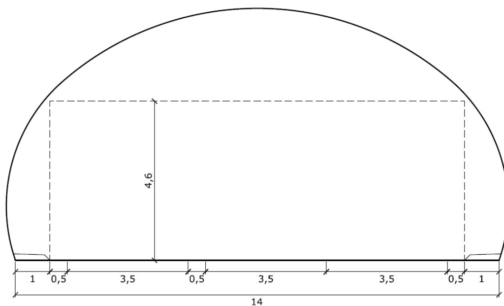
Figur V1.7 Tunnelprofil T14 med forsterket midtoppmerking og forbikjøringsfelt (mål i m).
