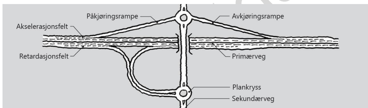
Figur D.18: Planskilt kryss – kryselementer
