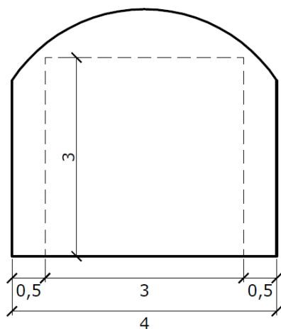
Figur V1.17 Tunnelprofil T4 (mål i m). T4 brukes for gang- og sykkelveger. T4 brukes for gangbare tverrforbindelser mellom tunnelløp og for nødutganger ut av tunnel
