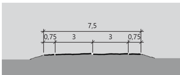
Figur C.8: Tverrprofil Hø2, vegbredde 7,5 (mål i m)
