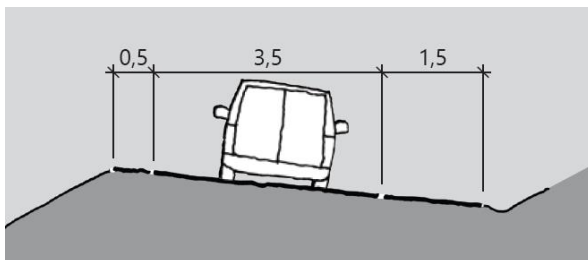
Figur D.19: Rampens tverrprofil (mål i m)
