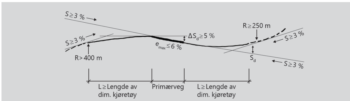
Figur D.2: Krav til sekundævegens vertikale linjeføring i kryssområdet
