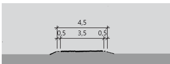
Figur C.7: Tverrprofil for Hø1, 1-feltsveg, vegbredde 4,5 (mål i m)
