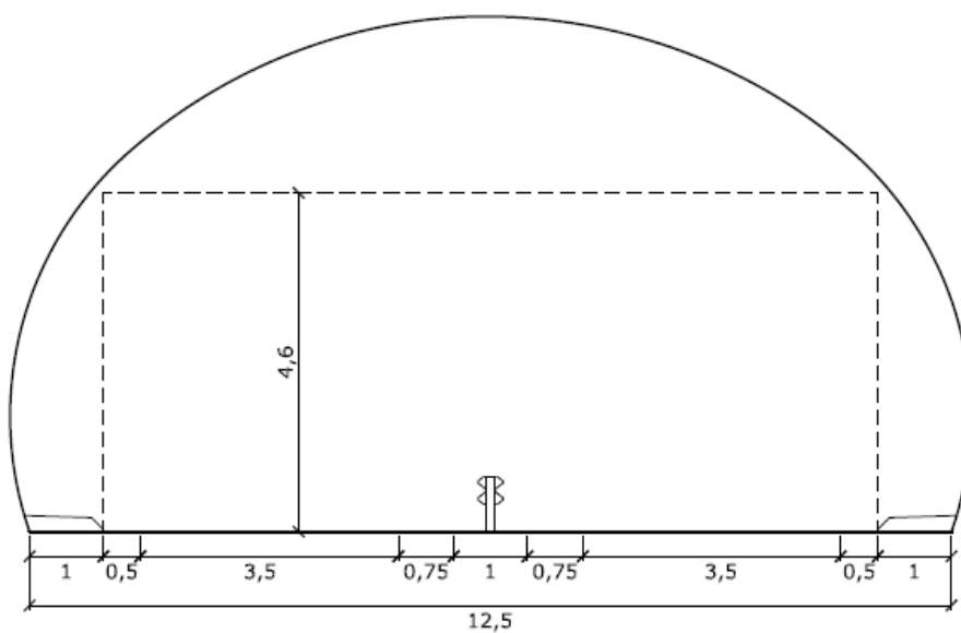
Figur V1.4 Tunnelprofil T12,5 med midtrekkverk (mål i m).
