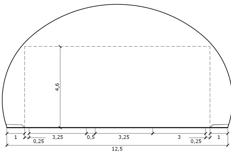
Figur V1.2 Tunnelprofil T12,5 med forsterket midtoppmerking og havarinisje (mål i m).
