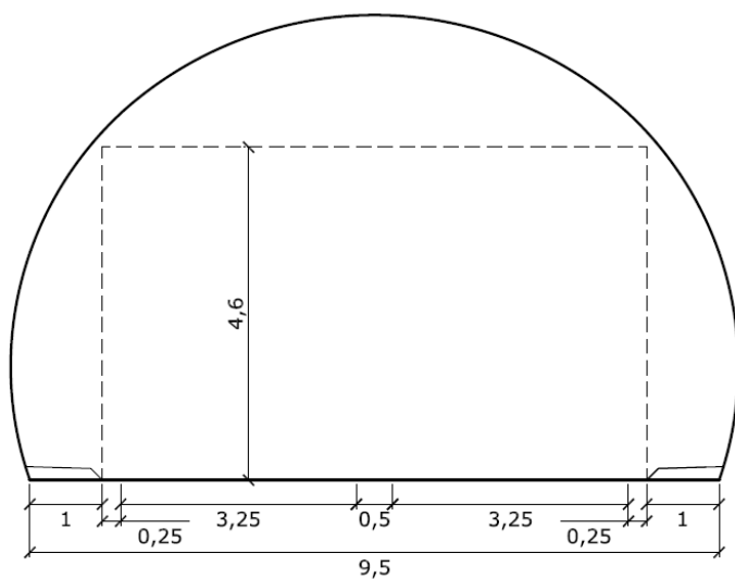
Figur V1.1 Tunnelprofil T9,5 med forsterket midtoppmerking (mål i m).
