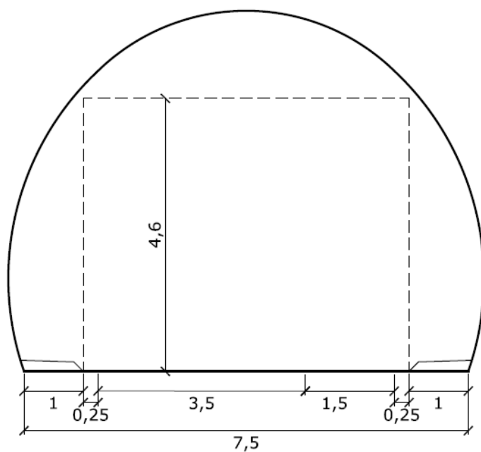
Figur V1.18 Tunnelprofil T7,5 (mål i m). Brukes for av- og påkjøringsramper med ett kjørefelt der havarert kjøretøy skal kunne plasseres.
