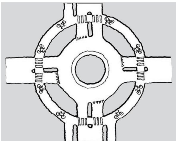
Figur D.14: Prinsippløsning for sykkel i rundkjøring, eksempel 2
