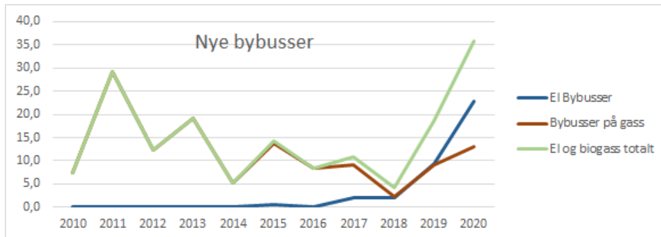
Figur 6: Registrerte bybusser i % per år fordelt på drivlinje (Kilde: Kjøretøyregisteret i SVV)
